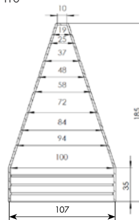
EPDM-Stufenmanschette für Flavent Dachdurchführungen DN 125
