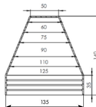
EPDM-Stufenmanschette für Flavent Dachdurchführungen DN 125
