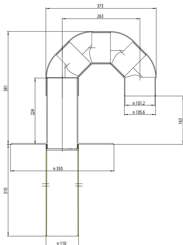
Dachdurchführungs-Set DN 110 mit Hart-PVC-Flansch
